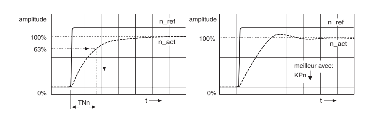
Illustration 7.13 Déterminer "TNn" en amortissement critique.
