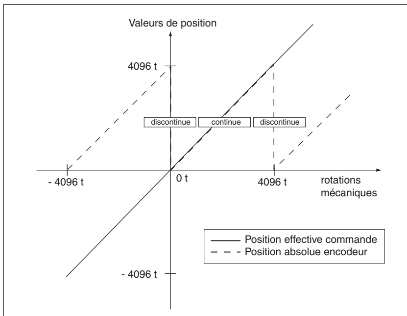
Illustration 7.10 Valeurs de position SinCos-Multiturn
