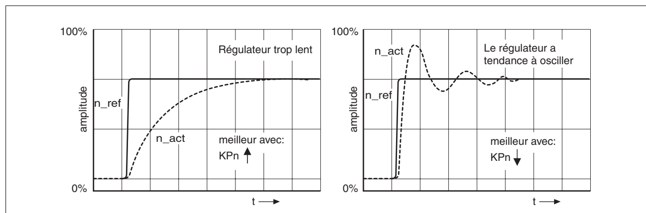
Illustration 7.15 Optimiser les réglages insuffisants du régulateur de vitesse de rotation
