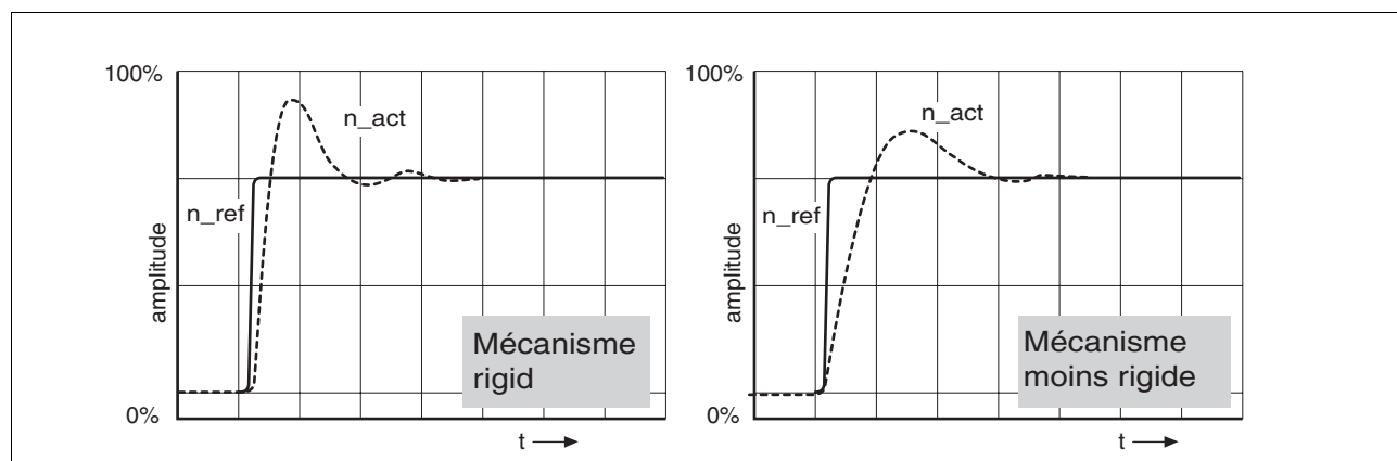
Illustration 7.14 Réponses de saut avec un bon comportement de régulation
