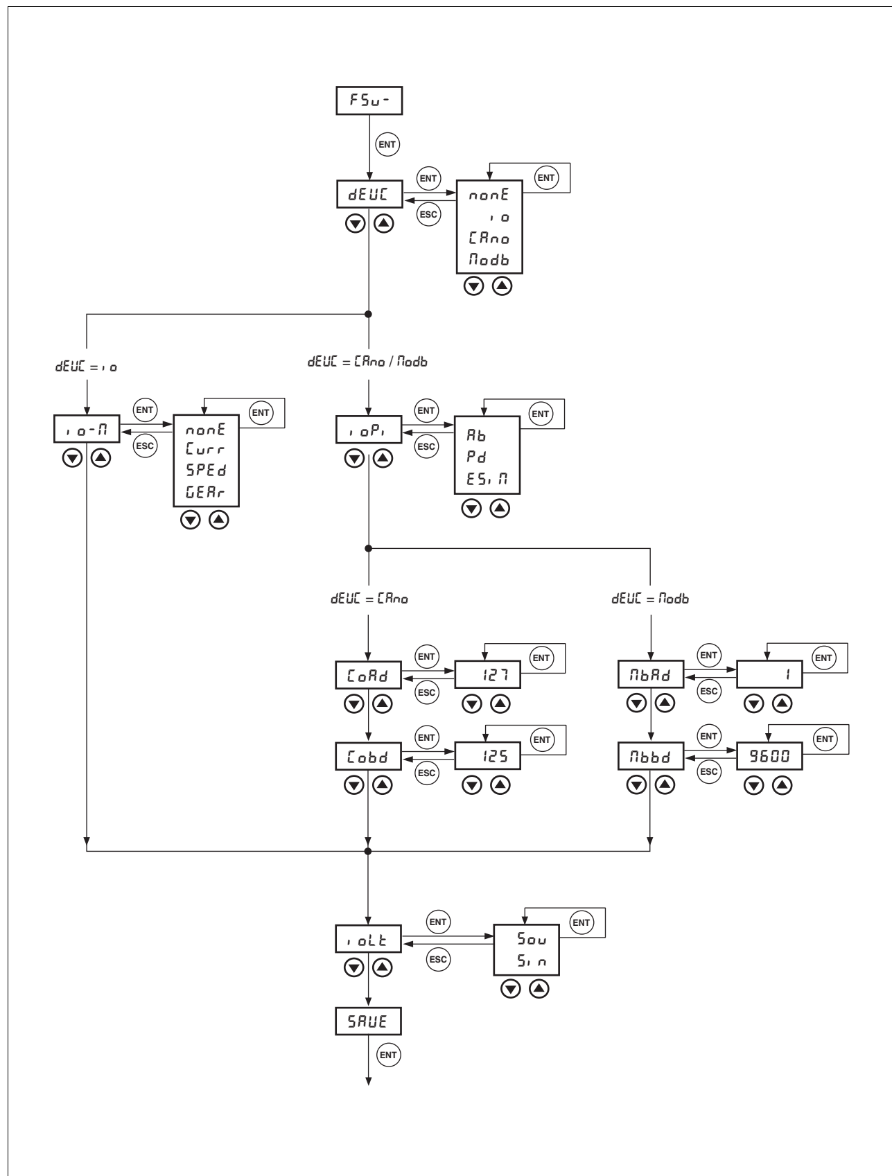
Illustration 7.6 "Première mise en service" à l'aide du panneau de commande HMI
