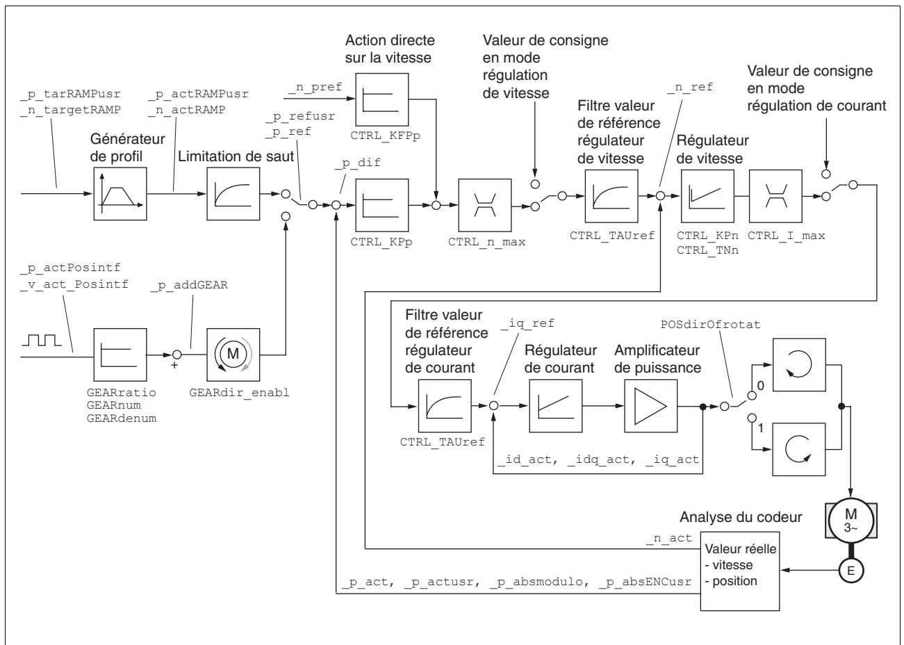
Illustration 7.11 Structure du régulateur pour l'évaluation du codeur via CN2
