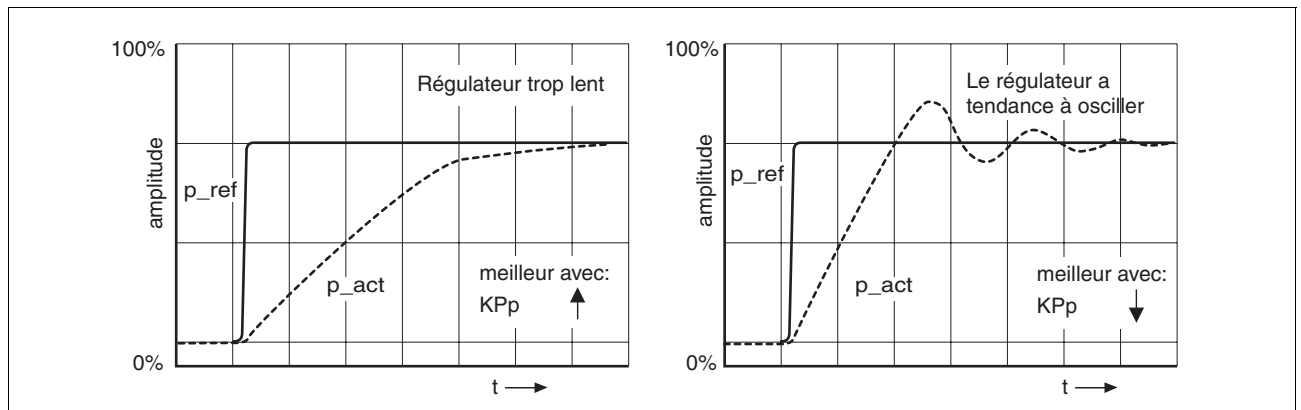
Illustration 7.17 Optimiser les réglages insuffisants du régulateur de positionnement
