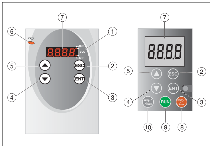
Illustration 7.2 HMI et terminal de commande déporté
