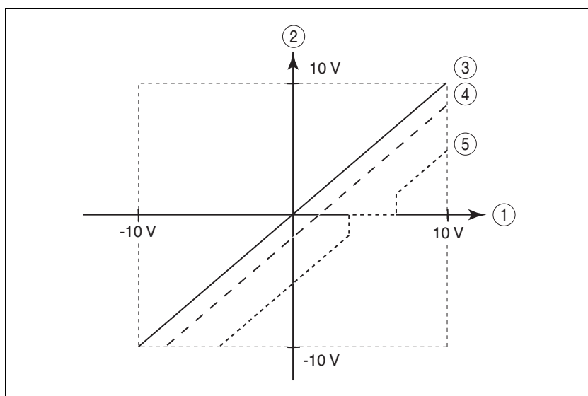
Illustration 7.8 Fenêtre offset et de tension nulle
