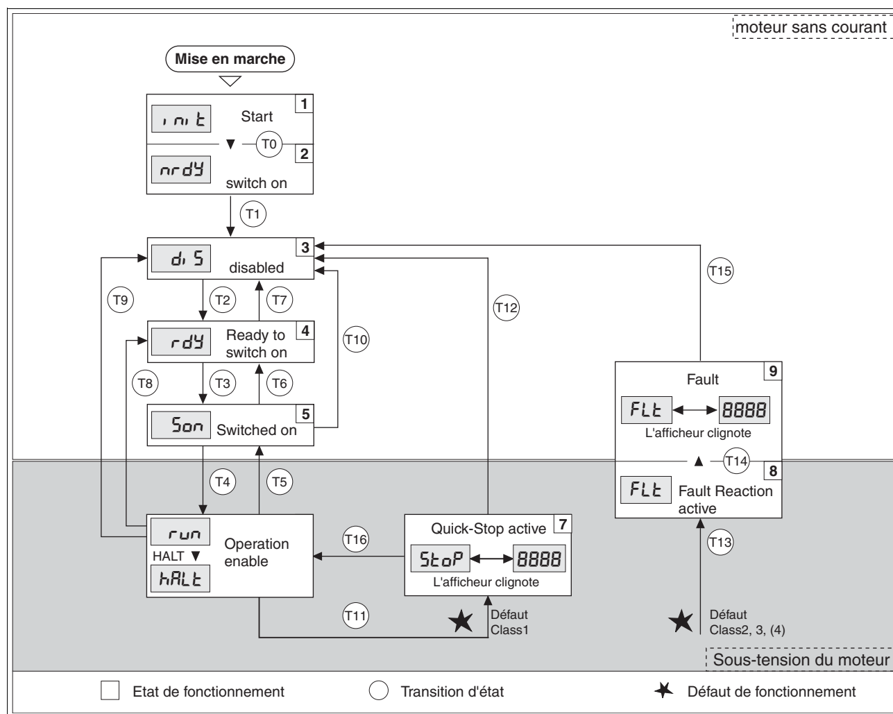
Illustration 7.7 Diagramme d'état
