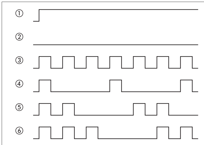
Illustration 7.3 Signification des signaux des LED
