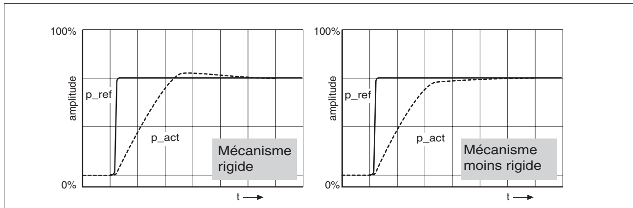
Illustration 7.16 Réponses de saut du régulateur de positionnement avec un bon comportement de régulation
