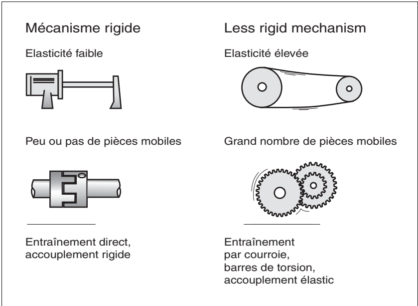
Illustration 7.12 Systèmes mécaniques à mécaniques rigide et moins rigide
